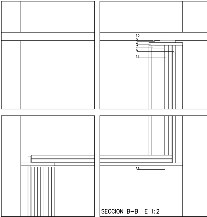
SECCION B-B E 1:2
