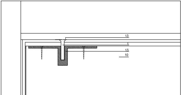
SECCION E-E E 1:2
