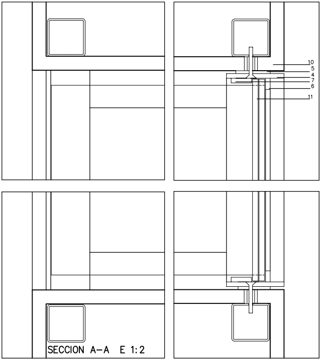
SECCION A-A E 1:2
