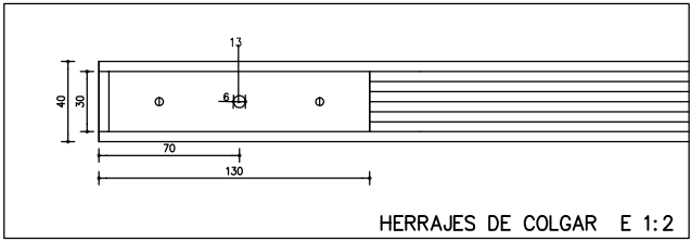
HERRAJES DE COLGAR E 1:2
