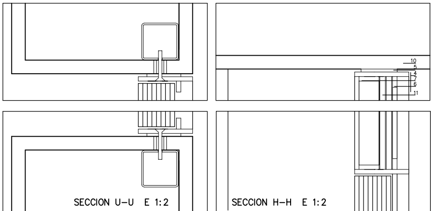
SECCION U-U E 1:2
